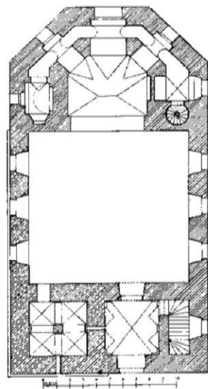
Obr. 197. Svobojín. Kostel sv. Petra a Pavla. Půdorys (bez hroby).
