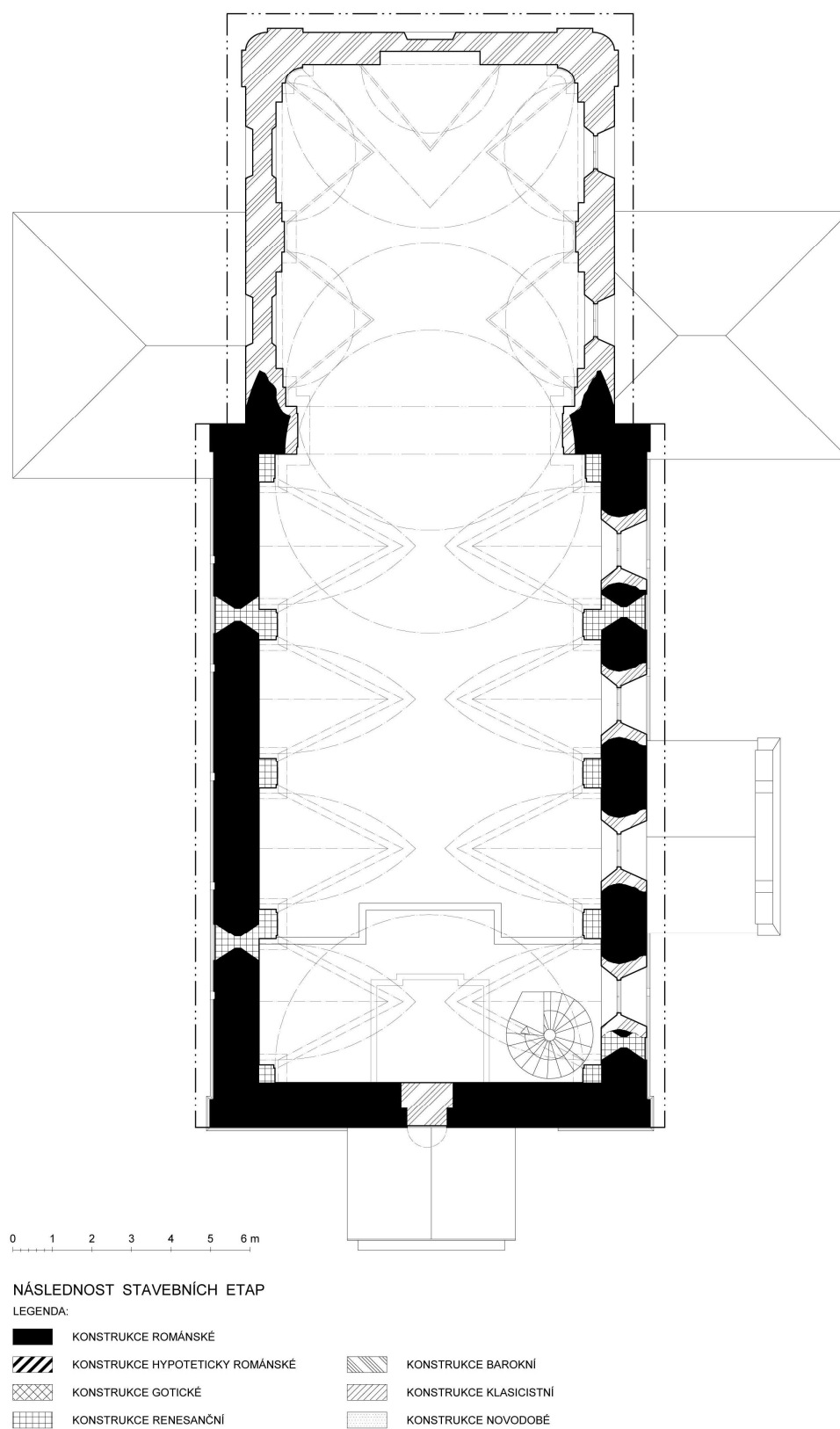
Obr. 4: Libčany (okr. Hradec Králové), kostel Nanebevzetí Panny Marie. Půdorys v úrovni empory s vyznačením stavebních fází (zaměření a kresba M. Falta 2006–2016).
