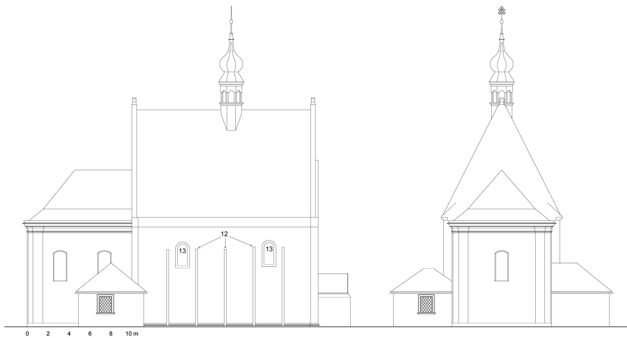
Obr. 7: Libčany (okr. Hradec Králové), kostel Nanebevzetí Panny Marie. Schéma severní a východní fasády s vyznačením určitých prvků: 12 – lizény zamýšleného (?) arkádového systému, 13 – zazděná románská okna (zaměření a kresba M. Falta 2006–2017).
