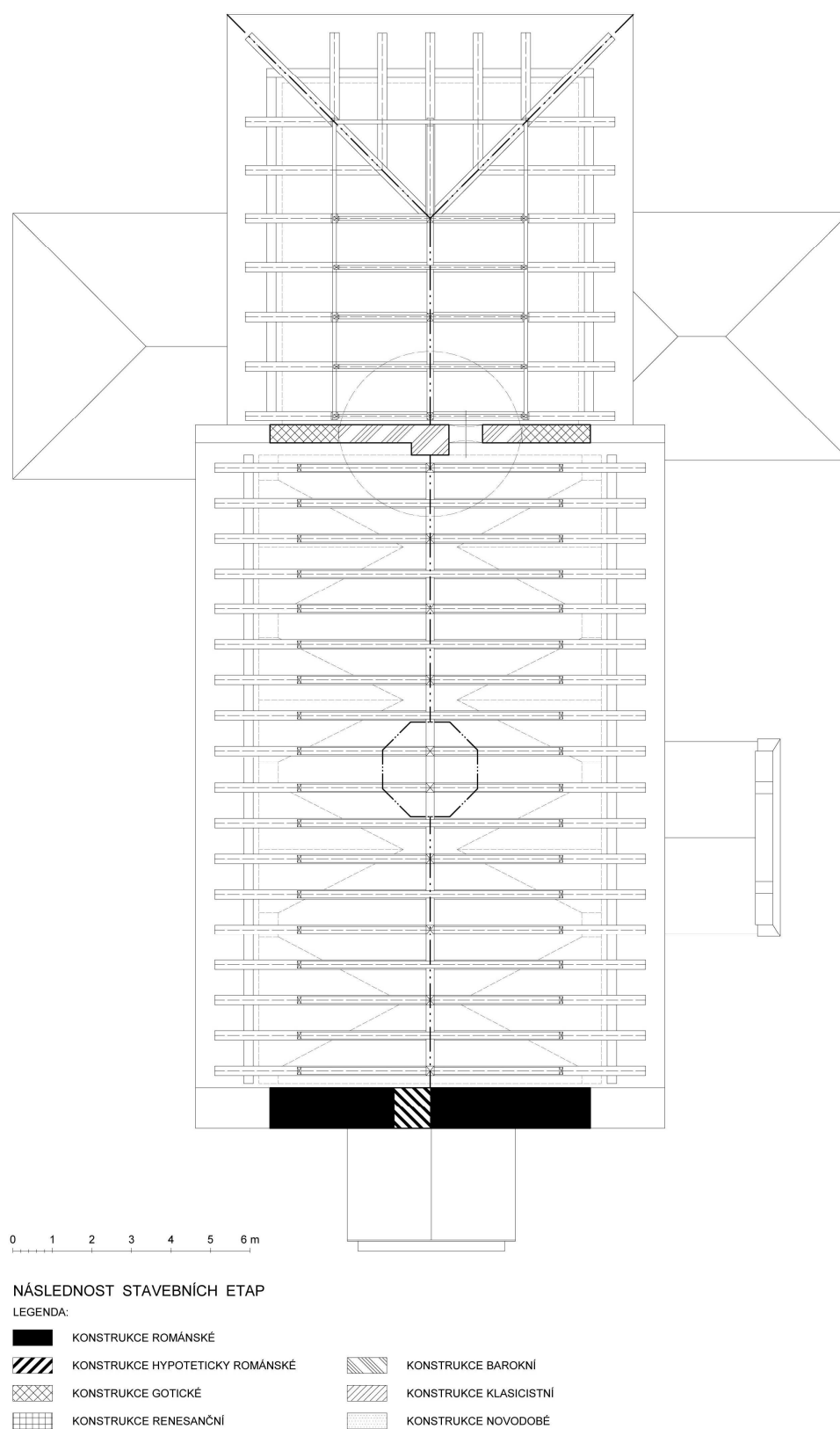
Obr. 5: Libčany (okr. Hradec Králové), kostel Nanebevzetí Panny Marie. Půdorys v úrovni krovu s vyznačením stavebních fází (zaměření a kresba M. Falta 2006–2016).
