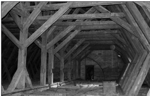
Obr. 19: Libčany (okr. Hradec Králové), kostel Nanebevzetí Panny Marie. Průhled renesančním krovem lodi směrem k východu (foto M. Falta 2006).
