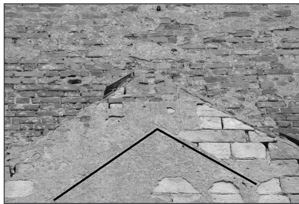
Obr. 17: Libčany (okr. Hradec Králové), kostel Nanebevzetí Panny Marie. Detail vrcholu románského štítu s pozůstatky omítky, která nese otisk střechy neznámé přisazené konstrukce. Stav v březnu 2005 – před opravou kostela (foto M. Falta 2005).
