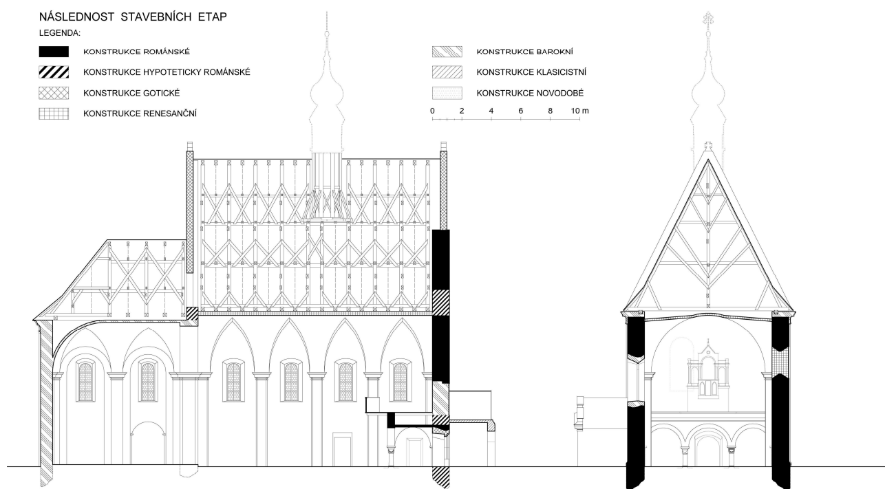
Obr. 8: Libčany (okr. Hradec Králové), kostel Nanebevzetí Panny Marie. Podélný a příčný řez (pohled k jihu, respektive západu) s vyznačením jednotlivých stavebních fází (zaměření a kresba M. Falta 2006–2016).
