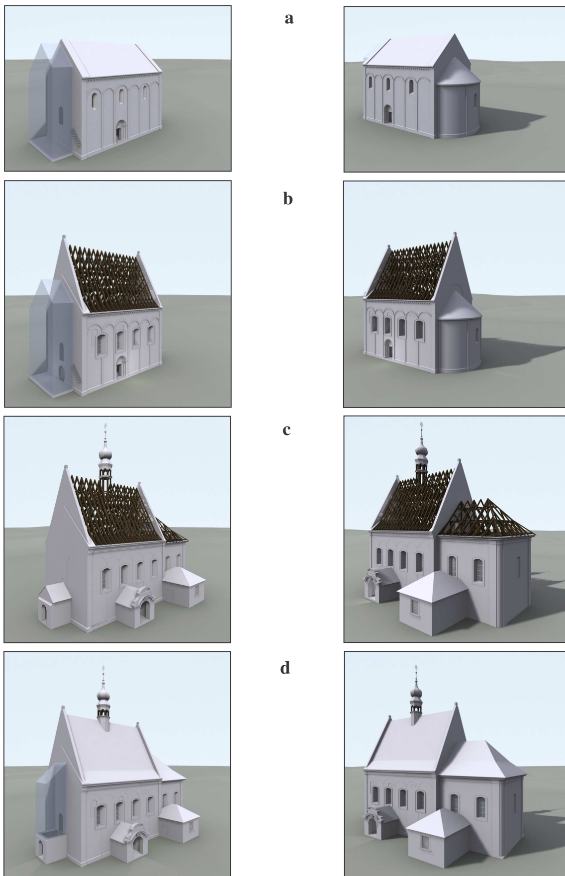
Obr. 10: Libčany (okr. Hradec Králové), kostel Nanebevzetí Panny Marie. 3D vizualizace kostela: a – možná románská podoba chrámu s naznačeným věžovým útvarem při západním průčelí, b – předpokládaná podoba chrámu na počátku 17. stol., c – podoba barokní přestavby kostela s vyznačeným renesančním krovem nad lodí a barokním nad chórem, d – současný stav objektu, průhledně zakreslena představa zaniklé novodobé věže (model M. Falta 2015–2017).
